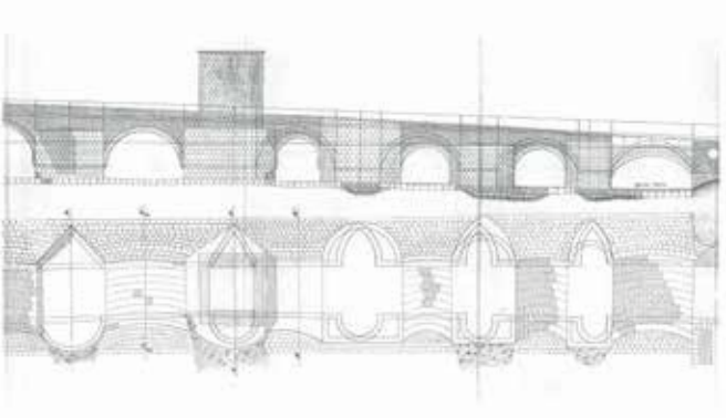
Alzado y planta del proyecto de reforma de 1908 en los últimos arcos, de E. Monterde; obsérvese la torre (en Ines Ingenieros Consultores, p. 106).
